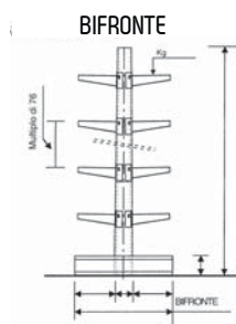
ESEMPIO CANTILEVER PER TUBI/PROFILI
