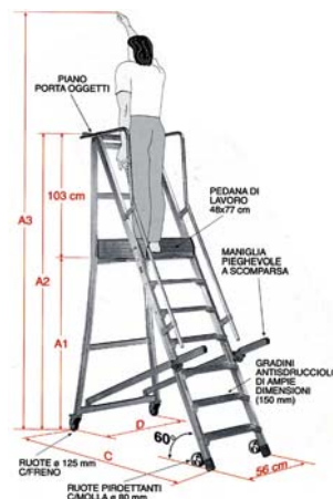
RUOTE CON FRENO
