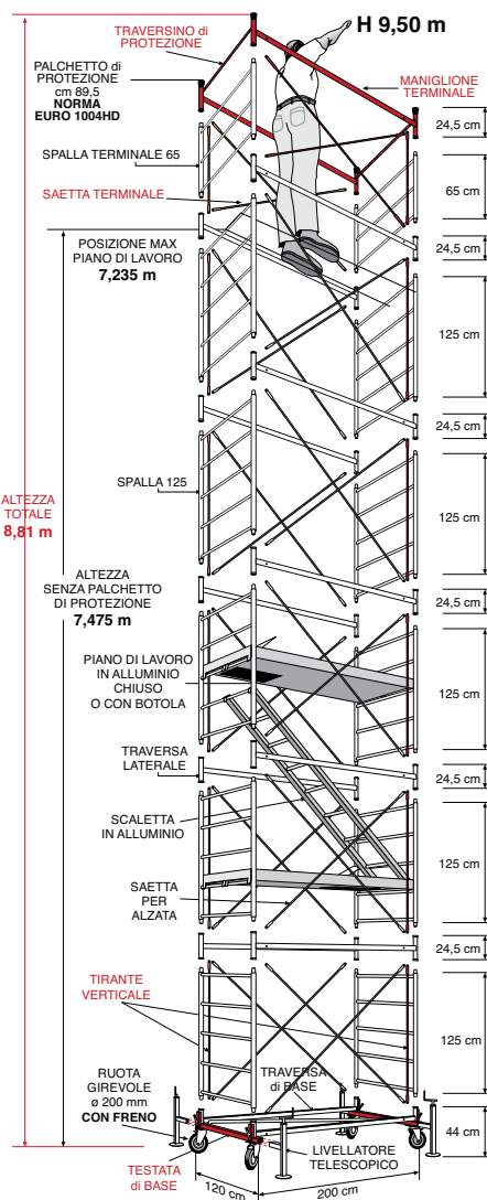
FTR 5 CON PIANO LAVORO E SCALA INTERNA
